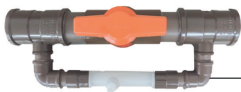
Conjunto venturi (injetor venturi + "bypass") Dimensões (C x L x A): 36,0 x 12,0 x 10,0 cm Peso: 0,8 kg
