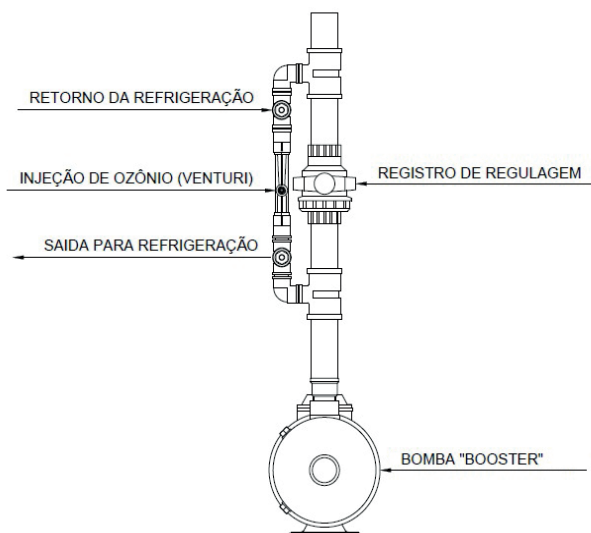
Conjunto "bomba booster" + venturi
