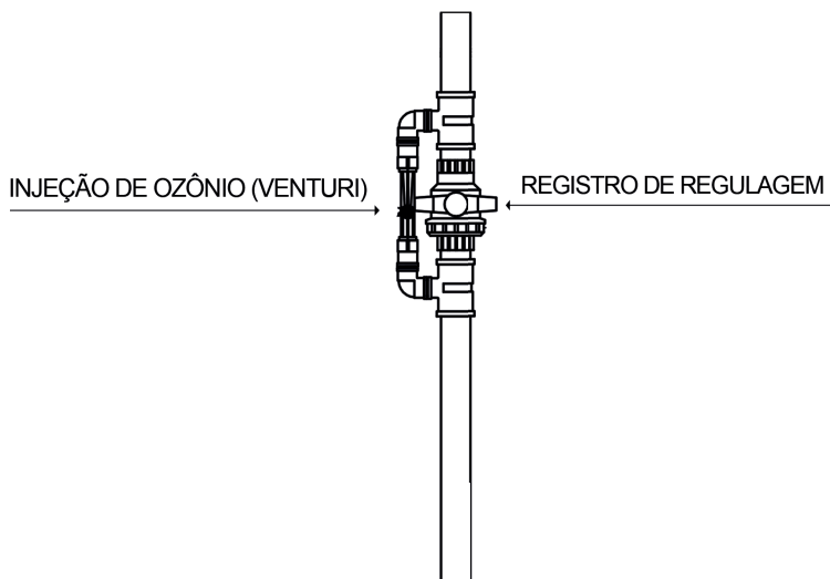
Conjunto venturi
