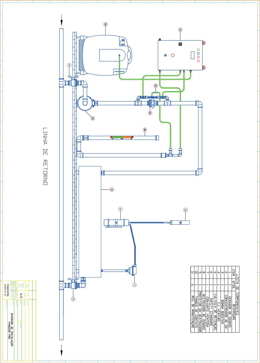
Tanque de contato instalado horizontalmente.
